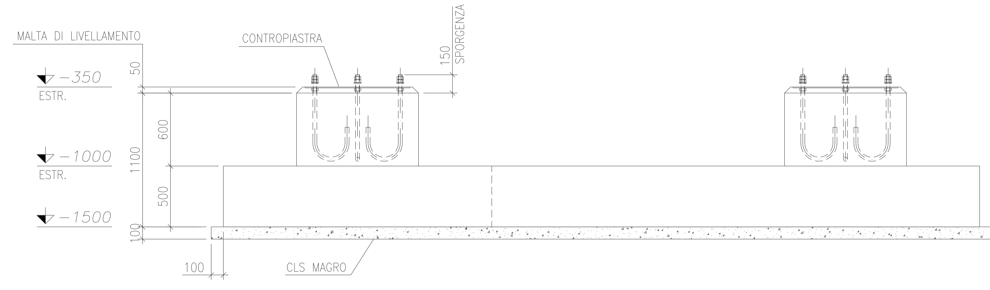
PLINTO TIPO "5" CASSEFORME 1:25
