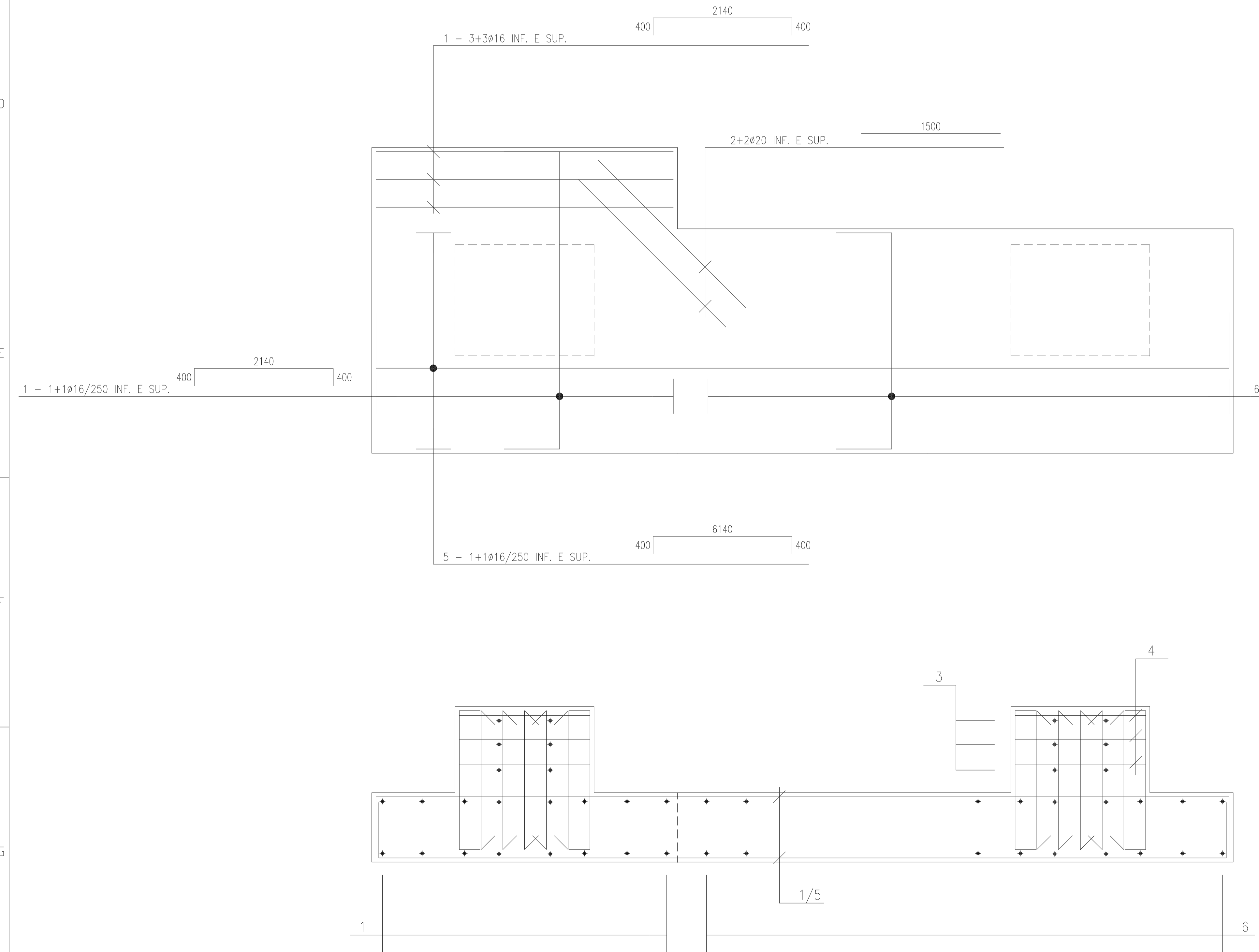
PLINTO TIPO "5" ARMATURA 1:25
