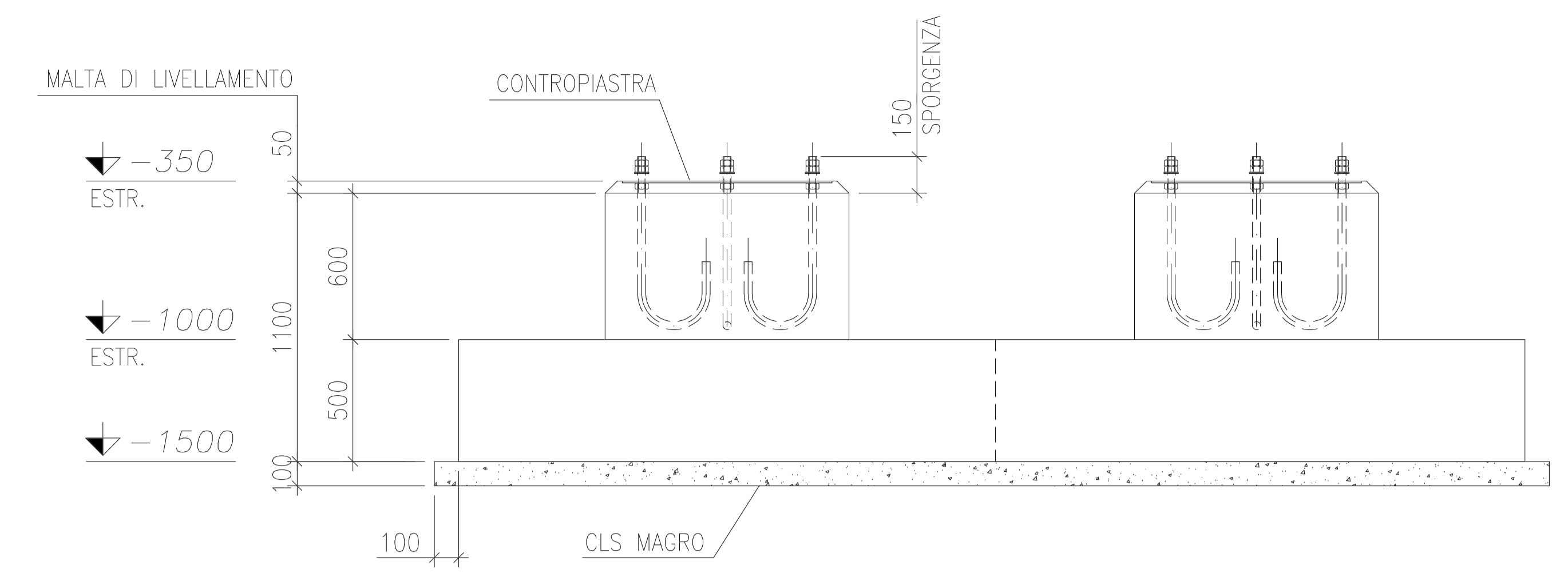
PLINTO TIPO "6" CASSEFORME 1:25
