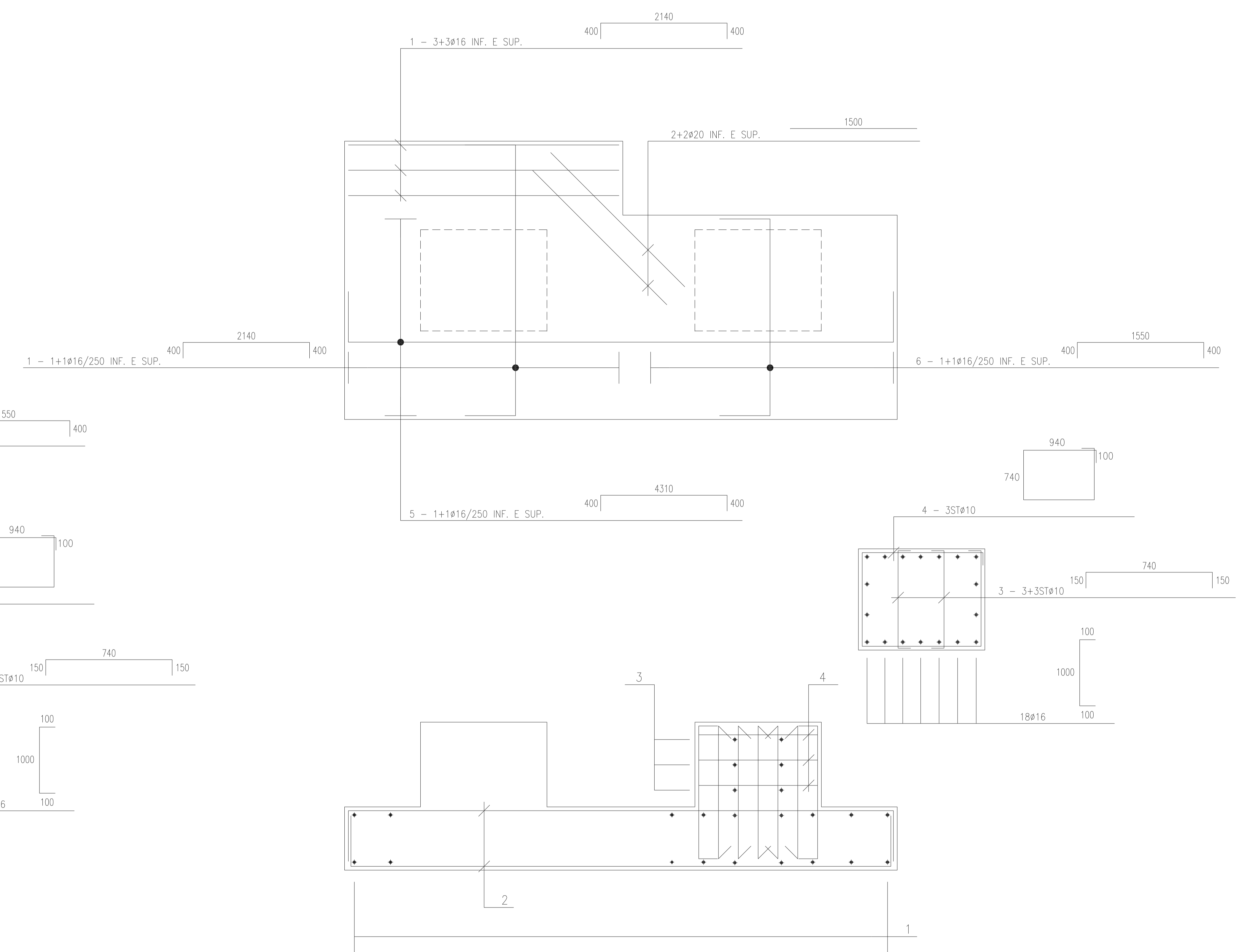
PLINTO TIPO "6" ARMATURA 1:25
